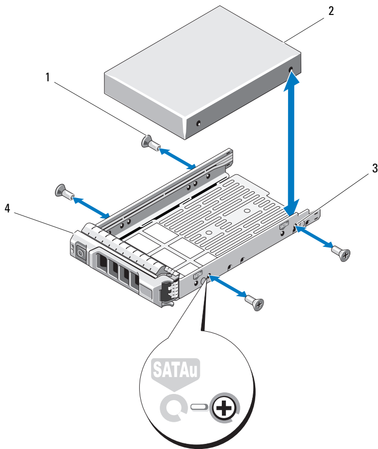
图 16-5. 卸除并安装硬盘驱动器到 3.5 英寸硬盘驱动器托盘中
